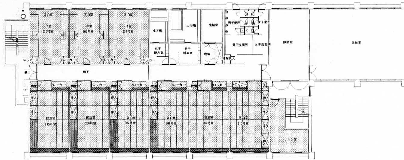
2階平面図
